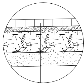
Przekrój konstrukcyjny zjazdu o nawierzchni z kostki betonowej
