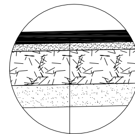
Przekrój konstrukcyjny zjazdu o nawierzchni bitumicznej
