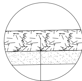
Przekrój konstrukcyjny zjazdu o nawierzchni z kruszywa łamanego
