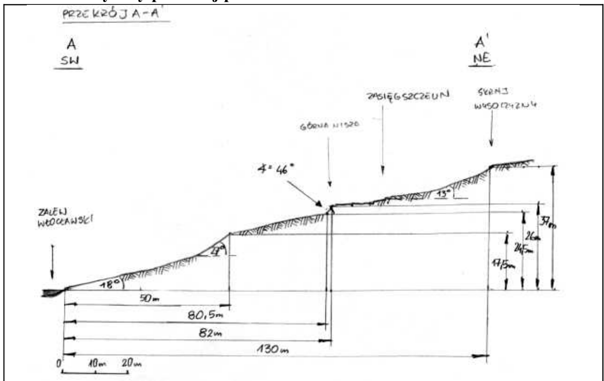
11. Schematyczny przekrój przez osuwisko
